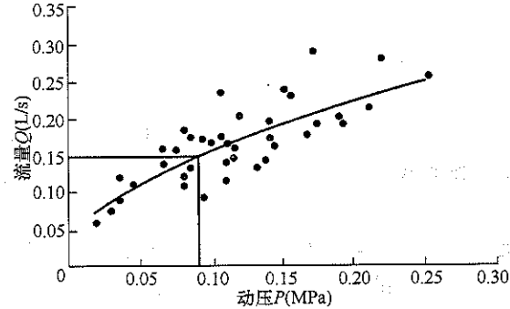
图 1 陶瓷阀芯水嘴半开 Q - P 曲线
